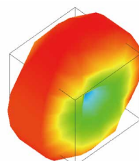
HFSSIによるRFID電波の3次元解析
